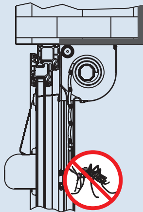
Prerez rolete z vgrajenim komarnikom
