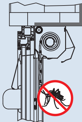
Prerez rolete z vgrajenim komarnikom
