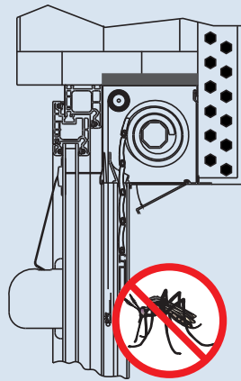
Prerez rolete z vgrajenim komarnikom
