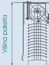
Montaža z 90° zglobom
